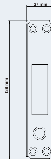
RECESS PLATE แผ่นรองฝัง
