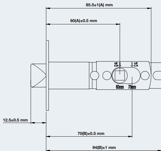
STANDARD TUBULAR LATCH ล็อกลูกสปริงมาตรฐาน
