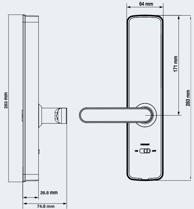
INDOOR UNIT โมดูลด้านในห้อง
