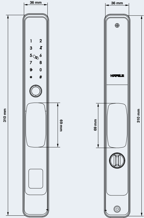
OUTDOOR UNIT โมดูลด้านนอกห้อง
