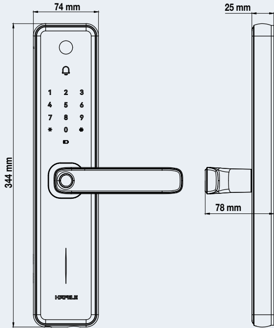
OUTDOOR UNIT โมดูลด้านนอกห้อง
