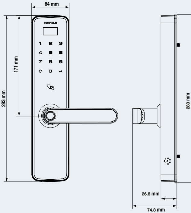
OUTDOOR UNIT โมดูลด้านนอกห้อง
