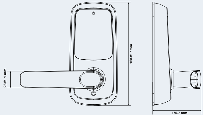
INDOOR UNIT โบลุด้านในห้อง
