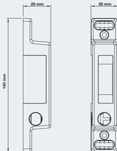
STRIKE PLATE เวนรับกลอน
