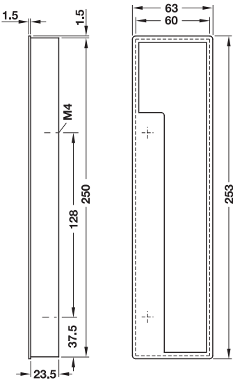
Handle for left hand door มือจับสำหรับด้านซ้ายของประตู
