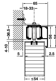
Wall installation with clip cover plate ติดตั้งบนผนัง สำหรับประตูบานไม้
