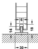
Floor guide without guide track in door leaf การติดตั้งกันแกว่งแบบไม่ใช้รางล่าง
