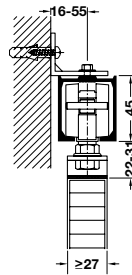
Wall installation with clip cover plate ติดตั้งบนผนัง สำหรับประตูบานไม้
