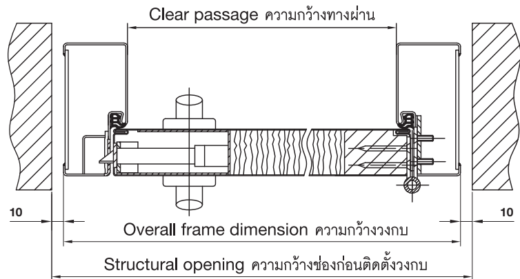
Flush door ประตูแบบเสมอวงกบ
