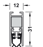
Double-side release ล้นสองด้าน
