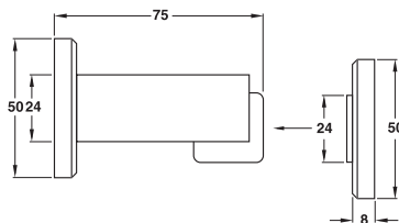
Wall mounted ติดตั้งกับผนัง
