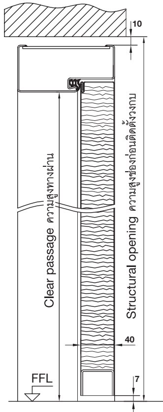
Flush door ประตูแบบเสมอวงกบ
