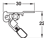
Maximum floor gap ความสูงจากพื้นถึงบานประตูสูงสุด
