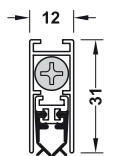
Single-side release ล้นด้านเดียว
